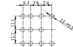
引出端形式：印制电路板式(P3) Terminal form: PCB(P3) MR20-1C/2C/3C-P3
