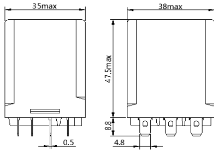
引出端形式(S2) Terminal style(S2) MR20-1C/2C/3C-S2
