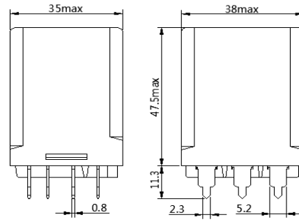
引出端形式：印制电路板式(P1) Terminal form: PCB(P1) MR20-1C/2C/3C-P1
